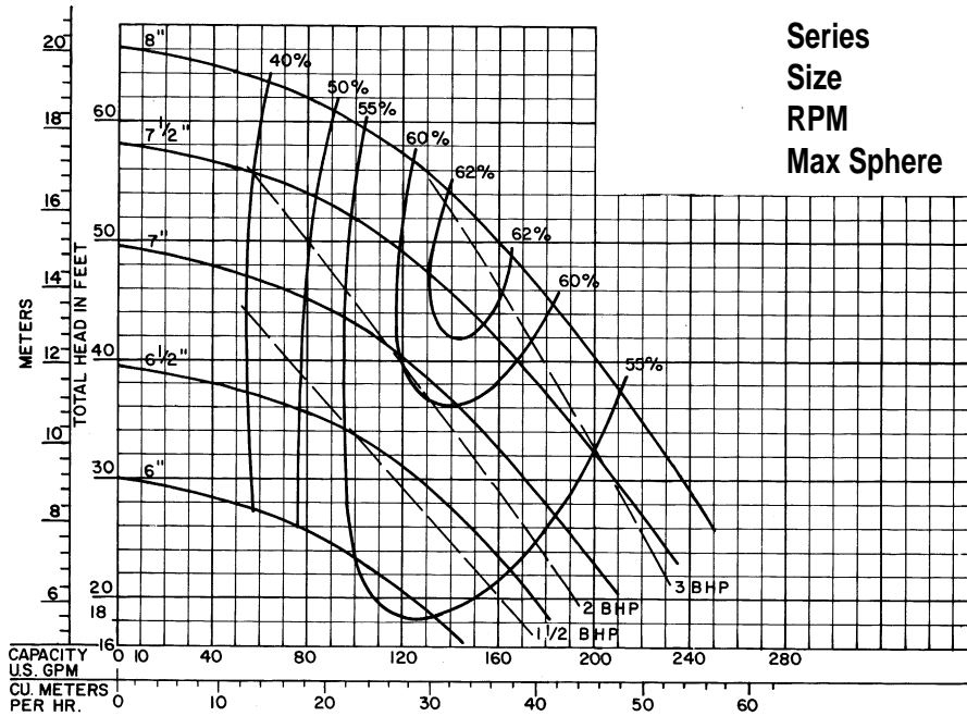
Curve CS-1620
